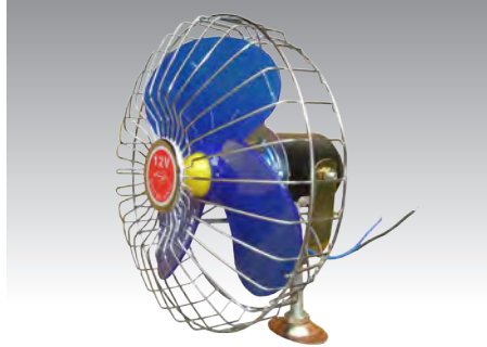
AUTO FAN CL-987 12V 16/4.9/20/22 CL-988 24V 16/4.9/20/22 CL-989 48V 16/6.0/22/24
